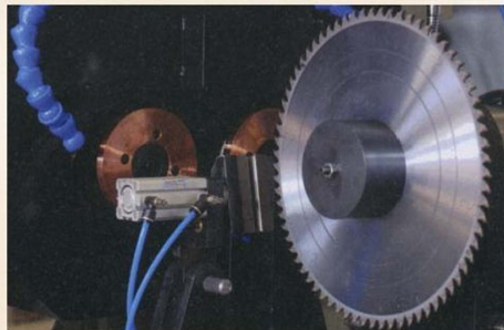
PCD齿侧刃双面同时加工
